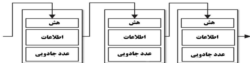
شکل ۱ ساختار زنجیره بلوکی یا بلاک چین (Gao et al. 2018)
